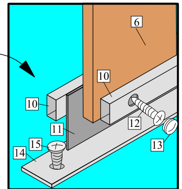
Oven alaosan rakenne Dörrrens nedre konstruktion
