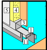
Vaihtoehto 1 Alternativ 1
