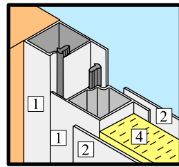
Tiiviste profiili Tättningsprofil
