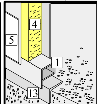
Vaihtoehto 3 Alternativ 3
