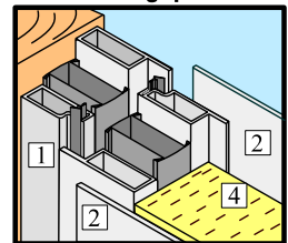
Kylmäkatkoprofiili Profil med köldspärr
